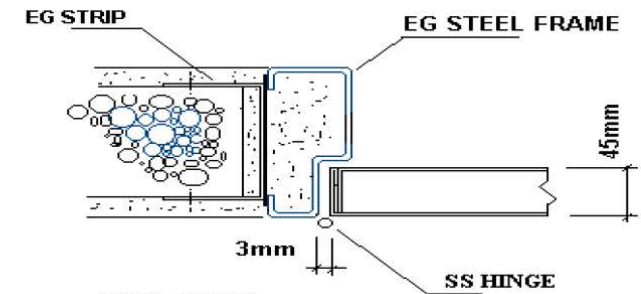
JAMB DETAIL
